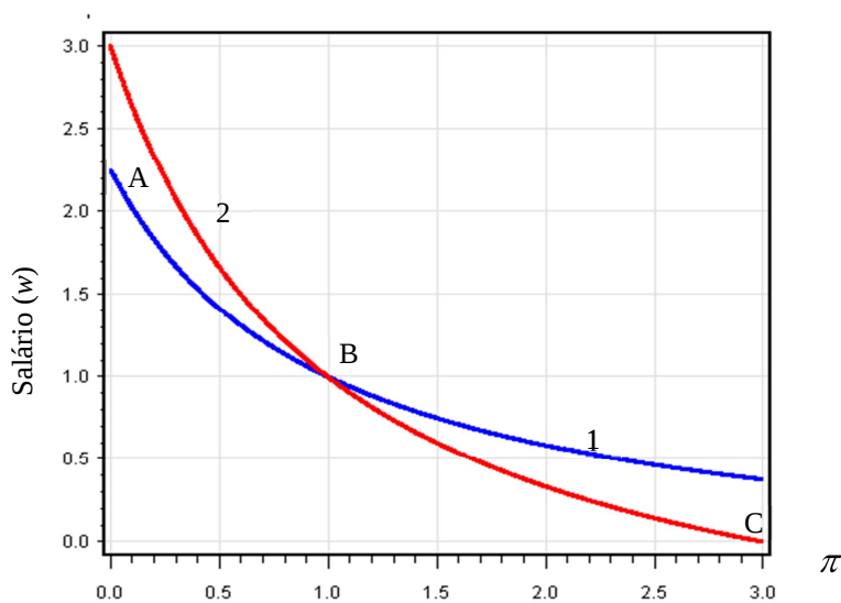
Figura 9. Relações w - \pi para o exemplo da Tabela 11
