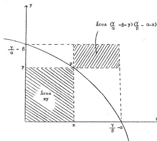
Figura 2. Arco de hipérbole côncavo.
