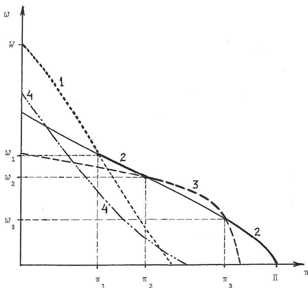
Figura 1. Relações w-\pi para quatro técnicas.
