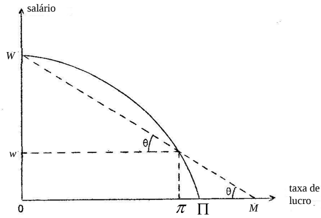
Figura 7. Determinação do valor do capital por unidade de trabalho ( k = \operatorname{tg} \theta ).
