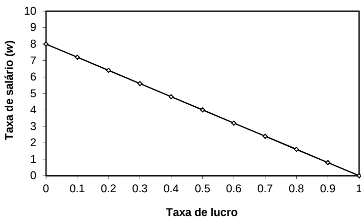
Figura 5. A fronteira tecnológica.
