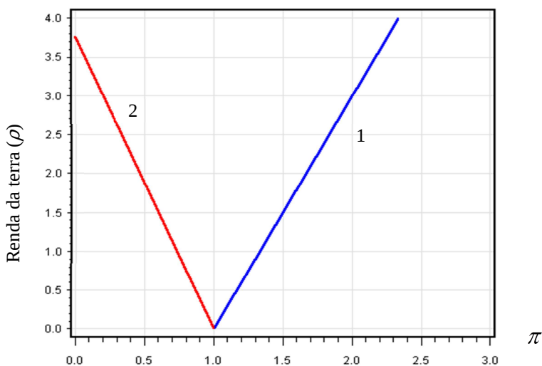
Figura 10. Variação da renda da terra em função de \pi para o exemplo da Tabela 11
