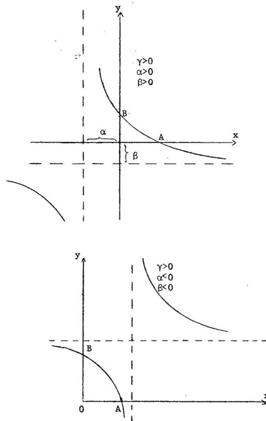
Figura 1. Arco de hipérbole convexo ou côncavo no primeiro quadrante.
