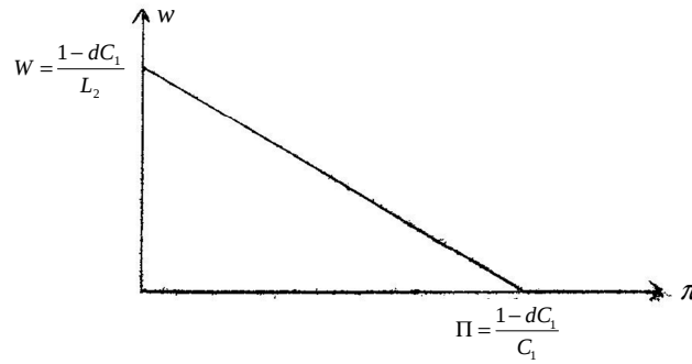
Figura 3. Relação w - \pi linear.
