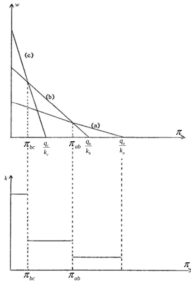
Figura 8. Relações w - \pi lineares e o respectivo valor do capital por unidade de trabalho ( k ).
