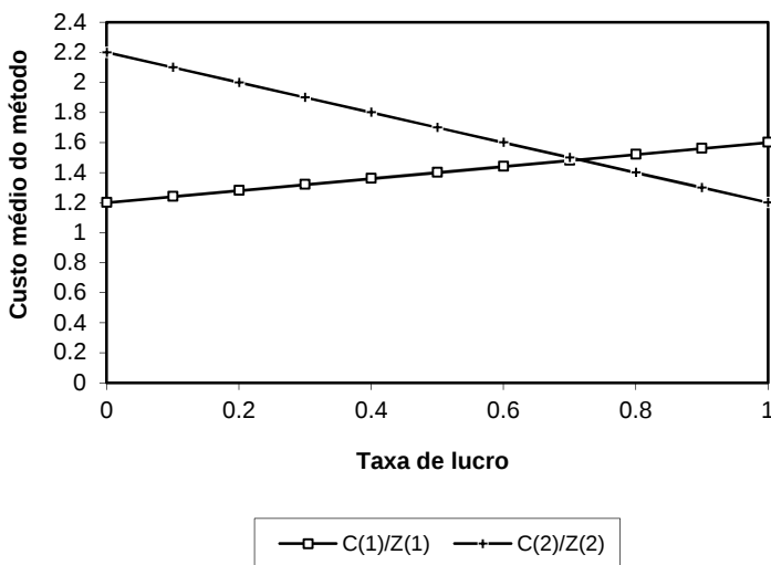
Figura 6. O comportamento dos custos médios.
