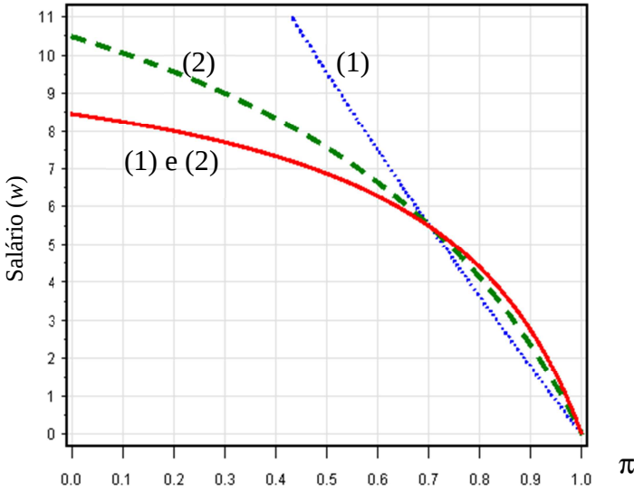
Figura 7. A renda intensiva e as mudanças autônomas na distribuição: curvas w - \pi
