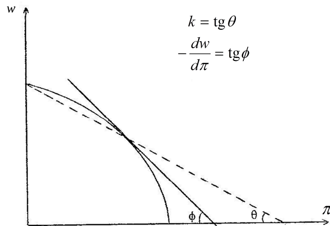
Figura 11. Determinação de k e de \frac{dw}{d\pi} em um ponto de uma relação w - \pi côncava.
