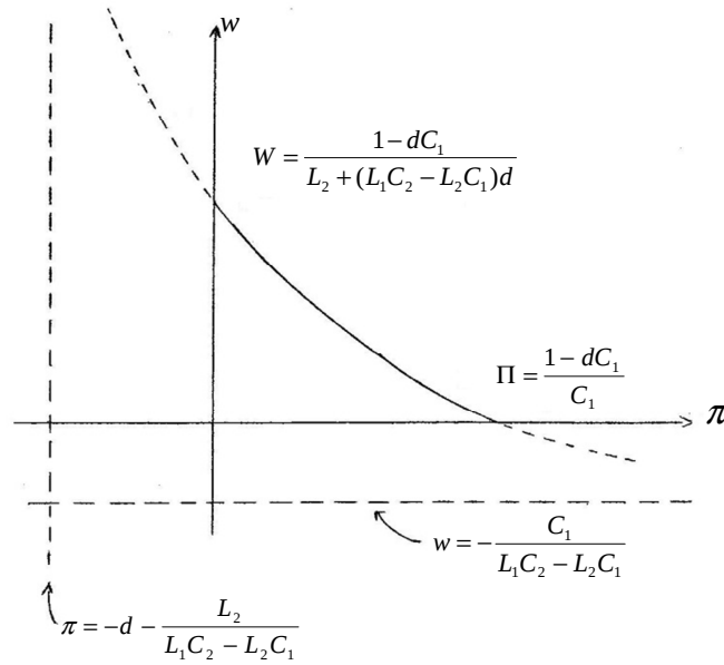
Figura 4. Relação w-\pi convexa.
