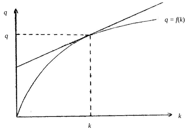
Figura 10. A função de produção agregada.
