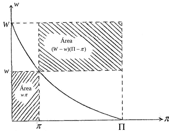
Figura 6. As áreas w\pi e (W - w)(\Pi - \pi) em uma relação w - \pi convexa.
