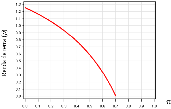
Figura 8. A renda intensiva e as mudanças autônomas na distribuição: curva \rho - \pi
