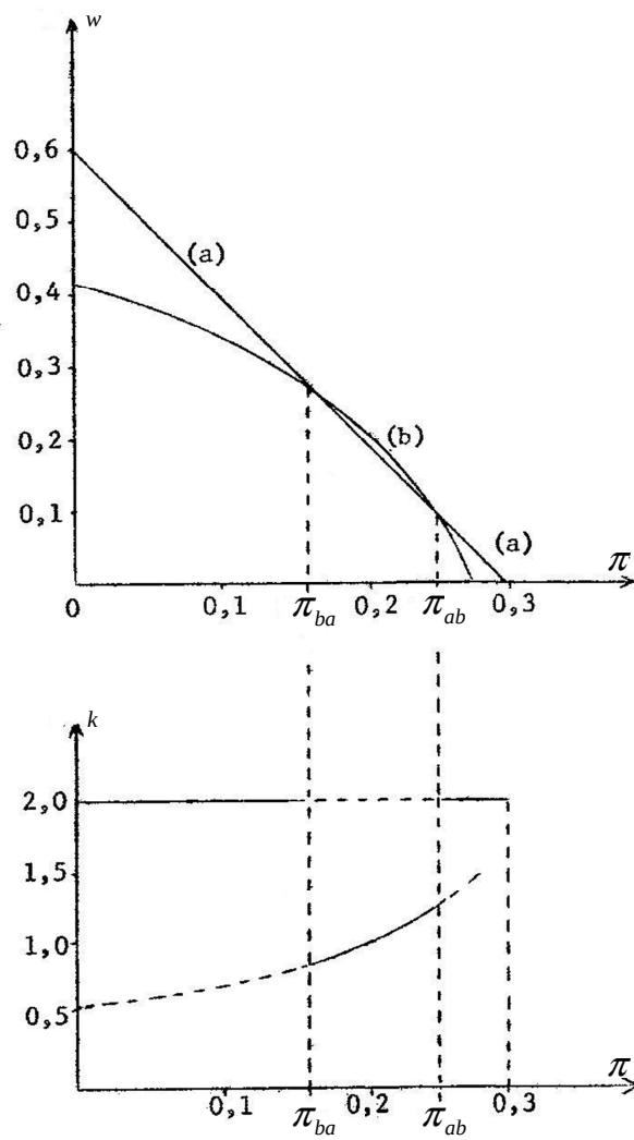
Figura 9. Duas relações w-\pi e as respectivas mudanças no valor do capital por unidade de trabalho ( k ).
