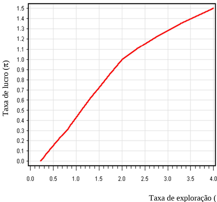
Figura 11. A taxa de lucro ( \pi ) como função da taxa de exploração ( \mu_1 ) para o exemplo da Tabela 11.
